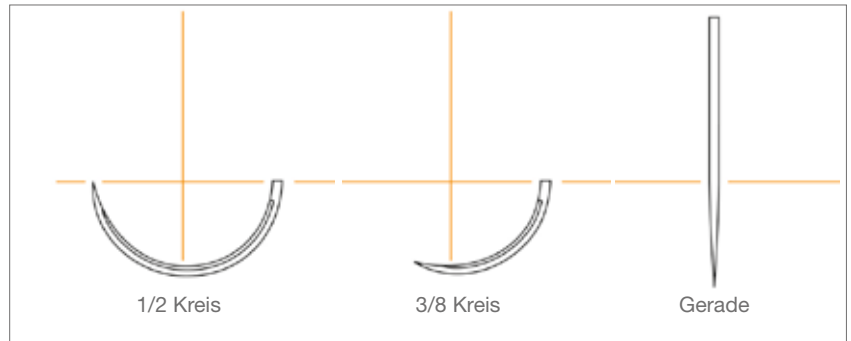
▲ Abb. 2: Nadeltypen
