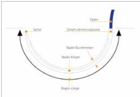
▲ Abb. 1: Nadelbeschreibung
